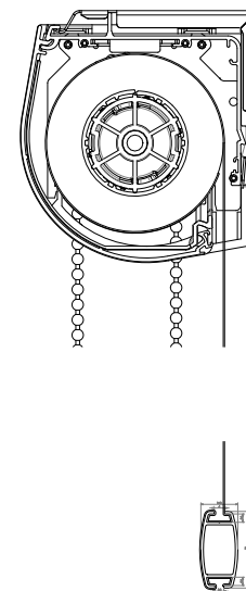
SECTION A-A
