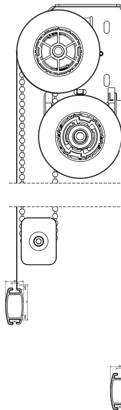
SECTION A-A
