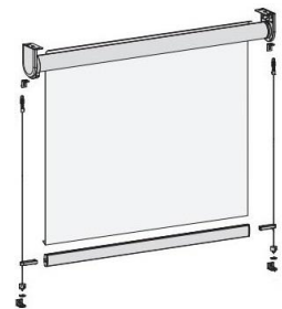
Σύστημα πλευρικών οδηγών συρματόσχοιου με επικάλυψη PVC
